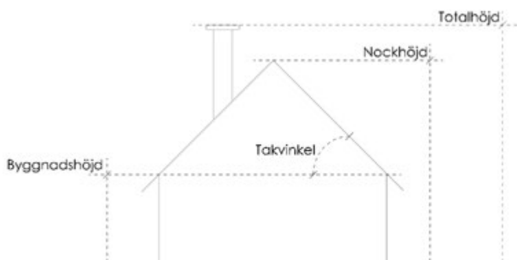
Illustration över vad som räknas som nockhöjd, byggnadshöjd och totalhöjd.
